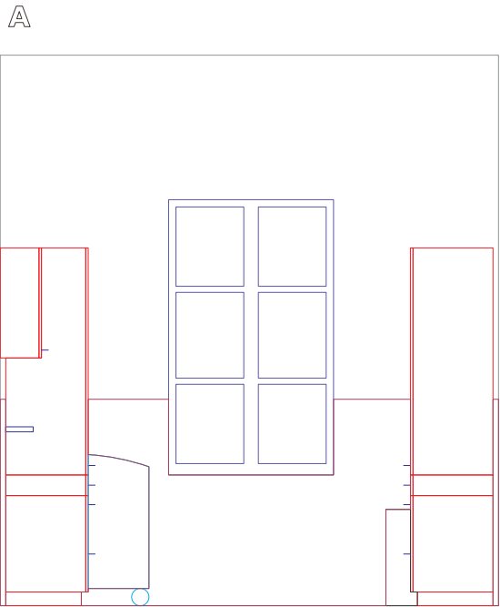
ŘEZ: UKÁZKA OBLOŽENÍ STĚN TL. 40mm V BAREVNÉM PROVEDENÍ
